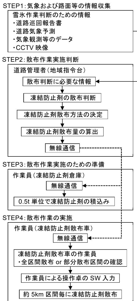
図 2.1 既存の凍結防止剤の散布方法のフロー
