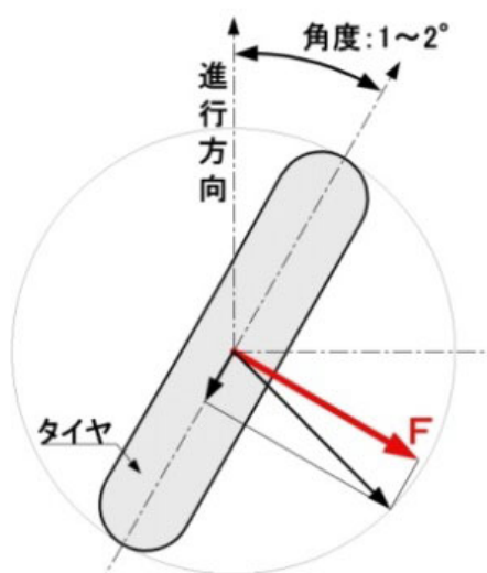
図 1.21 連続路面すべり抵抗値測定装置 (CFT) 外観 (左) と測定概念図 (右)
