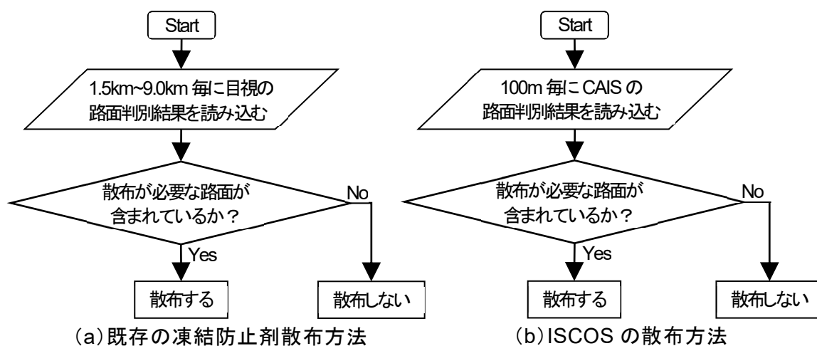
図 4.7 既存の散布方法と ISCOS の比較
