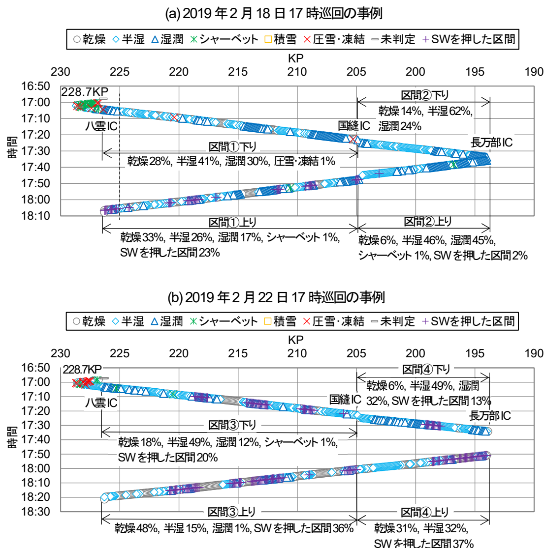
図 5.5 2019 年 2 月 18 日 17 時と 2019 年 2 月 22 日 17 時に八雲 IC～国縫 IC および国縫 IC～長万部 IC の路線の路面判別結果(路面判別結果をもとに 100m 区間散布を行った事例)
