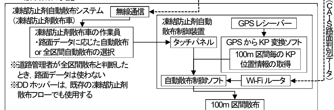
図 4.1 ISCOS による凍結防止剤散布フロー
