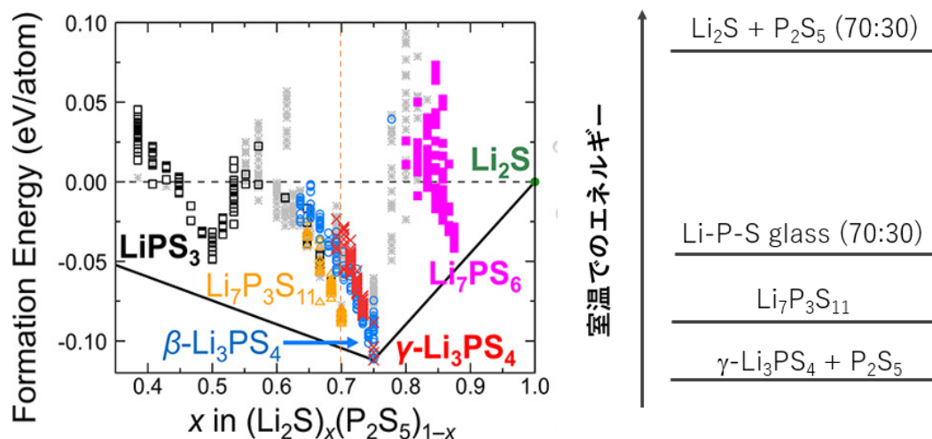
図2 (左) \text{Li}_2\text{S} と \text{P}_2\text{S}_5 の熱力学的凸包 (Convex hull). [5]. 結晶相にとさまざまなガラスを模した局所構造エネルギーを計算で示している. (右) 室温における \text{Li}_3\text{PS}_4\text{:P}_2\text{S}_5 の比を 70:30 とした際のエネルギー単位.
