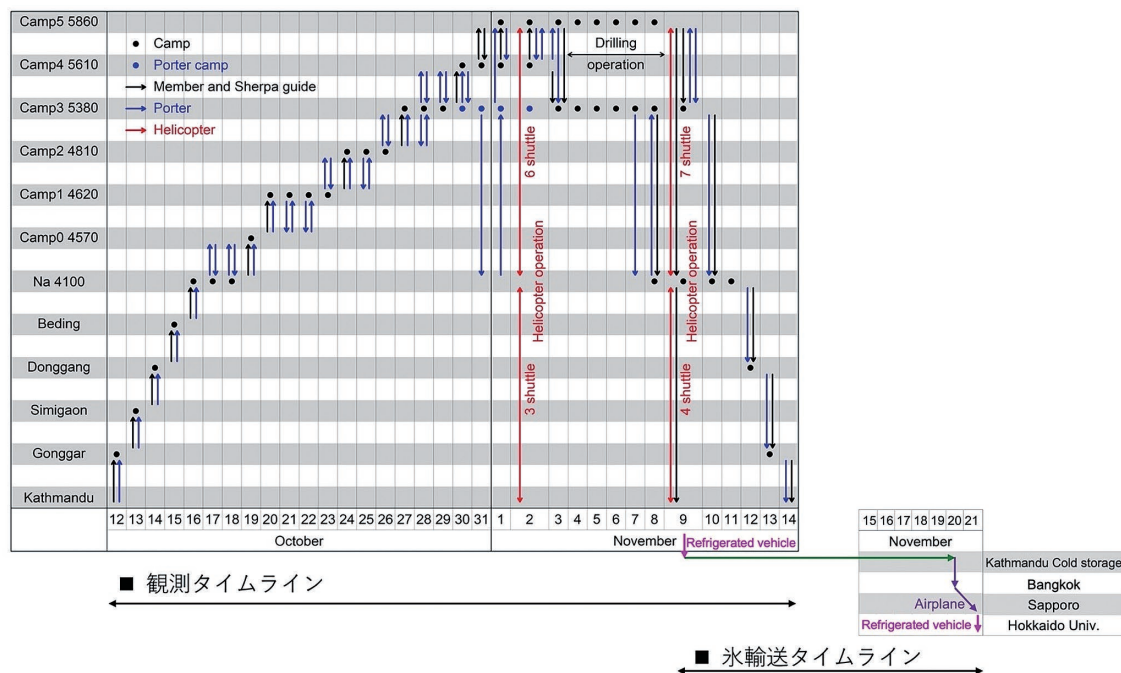
図3：アイスコア掘削を含むヒマラヤ氷河観測のタイムラインと氷輸送のタイムラインを示した。キャンプの標高(海抜表記)を併せて示した。Tsushima et al. (2021)に加筆。
