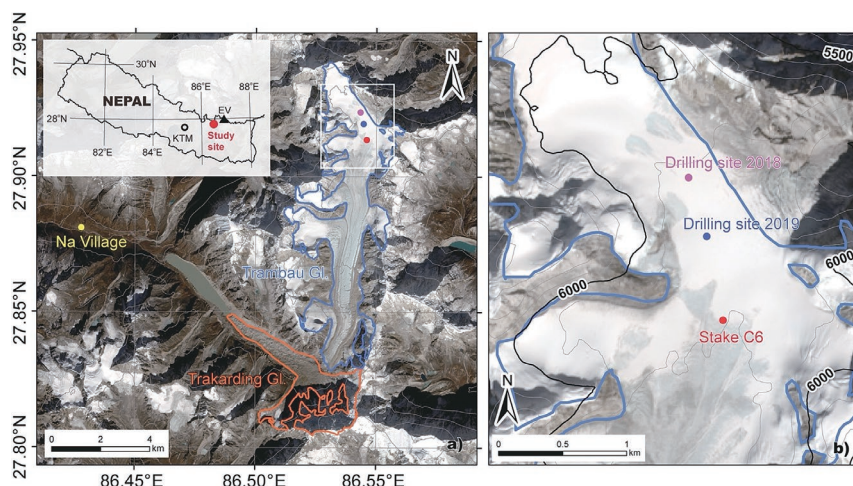
図1：(a)ネパール・ヒマラヤ、ロールワリン地域にあるトラカルディンートランバウ氷河の概要。左上にはロールワリン地域(赤丸)、カトマンズ(KTM)、およびエベレスト(EV)の位置関係を示した。黄色の丸で示したNa村は、標高4,100 mに位置し、氷河にアクセスする前に通る最後の村である。(b)掘削地点の拡大図を示した。氷河の境界は、GAMDAM氷河インベントリ(Nuimura et al., 2015; Sakai, 2019)で補正した。背景の氷河の画像は、2017年11月24日に撮影されたセンチネル2の衛星画像である。Tsushima et al. (2021)より引用。
