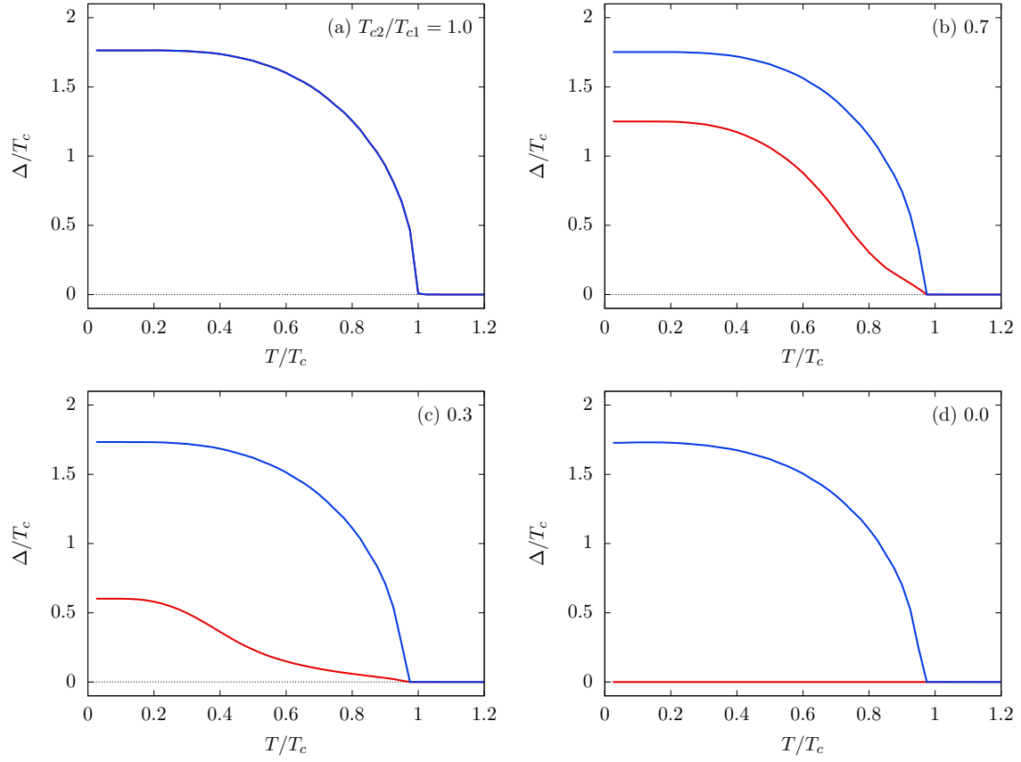
図 3.4 自己無撞着に計算した各バンドのペアポテンシャルの温度依存性. 青が \Delta_1 を, 赤が \Delta_2 を表す.
