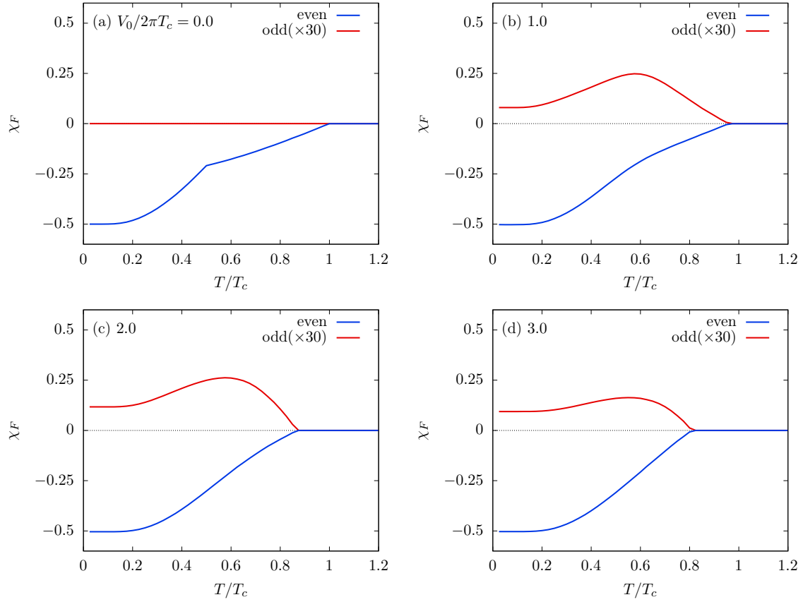
図 3.3 スピン磁化率に対する偶周波数成分・奇周波数成分の寄与。青が偶周波数成分からの寄与，赤が奇周波数成分からの寄与を表す。ただし，見やすいように奇周波数成分の寄与は 30 倍の値をプロットしている。
