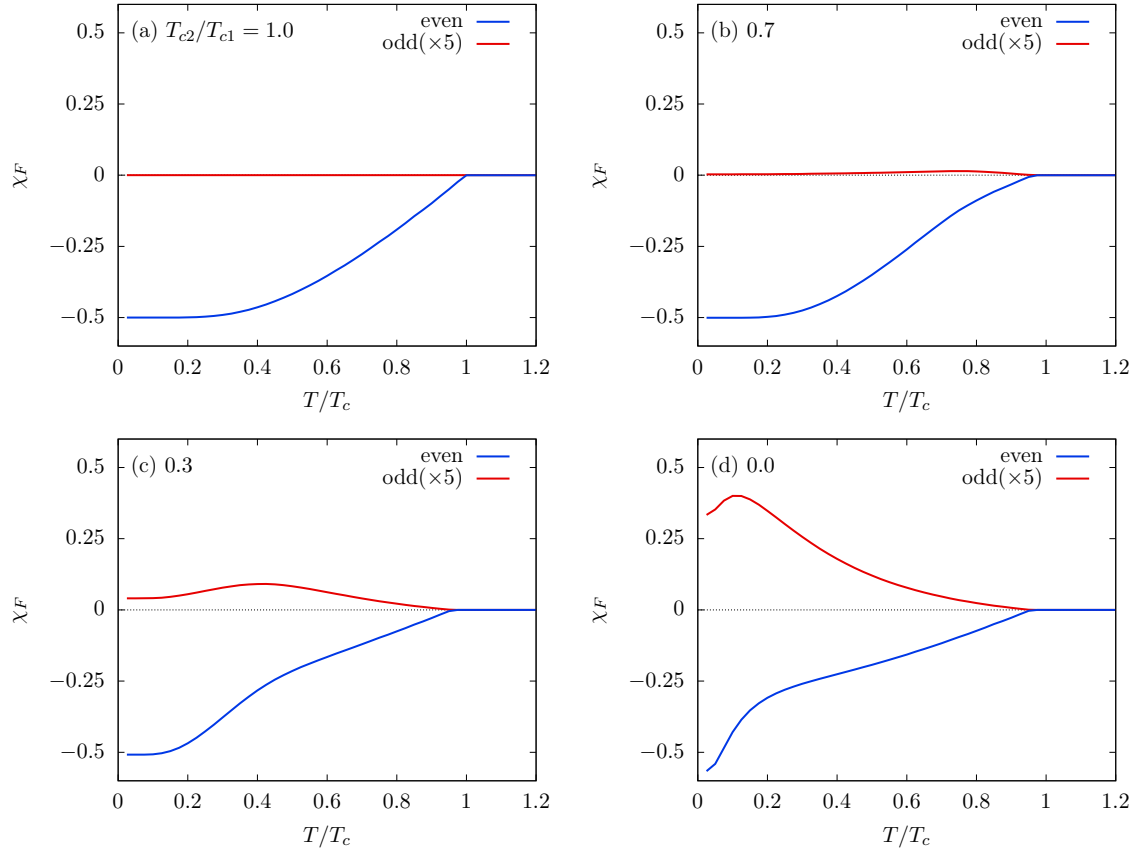
図 3.6 スピン磁化率に対する偶周波数成分・奇周波数成分の寄与。青が偶周波数成分からの寄与、赤が奇周波数成分からの寄与を表す。ただし、見やすいように奇周波数成分の寄与は 5 倍の値をプロットしている。
