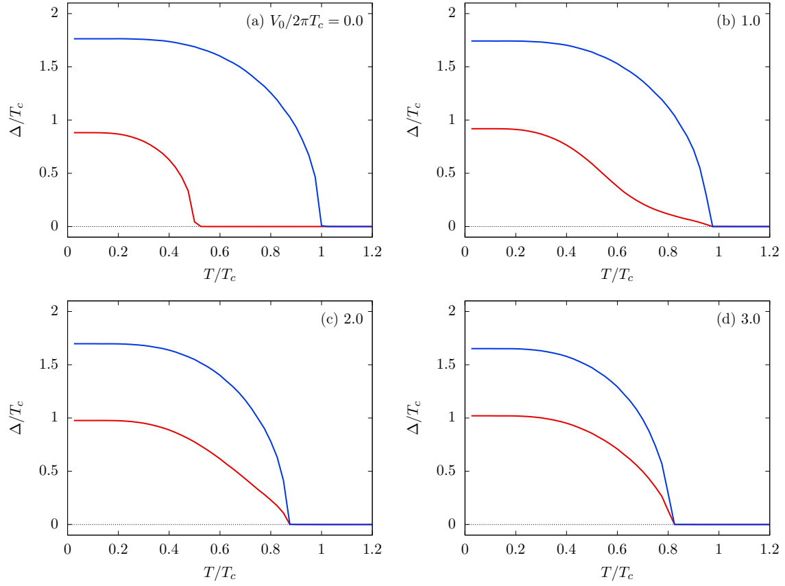
図 3.1 自己無撞着に計算した各バンドのペアポテンシャルの温度依存性. 青が \Delta_1 を, 赤が \Delta_2 を表す.
