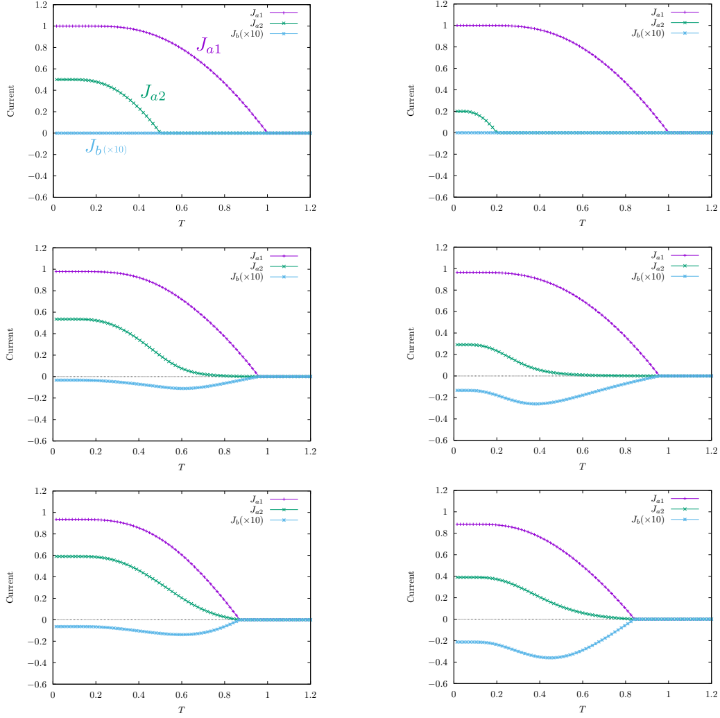
図 4.3 ジョセフソン電流の各成分を温度の関数として示した．超伝導体のパラメータ ( T_{c1}, T_{c2}, |V_0| ) は左右で等しくとり， V_0 = 0 における二つのバンドの転移温度が，左列は T_{c1}/T_{c2} = 0.5 ，右列は T_{c1}/T_{c2} = 0.2 となっている．またどちらの列も上から順に |V_0| = 0, |V_0| = 0.1, |V_0| = 0.2 のように混成項の大きさを大きくしている．ただし J_b については 10 倍した値をプロットしている．
