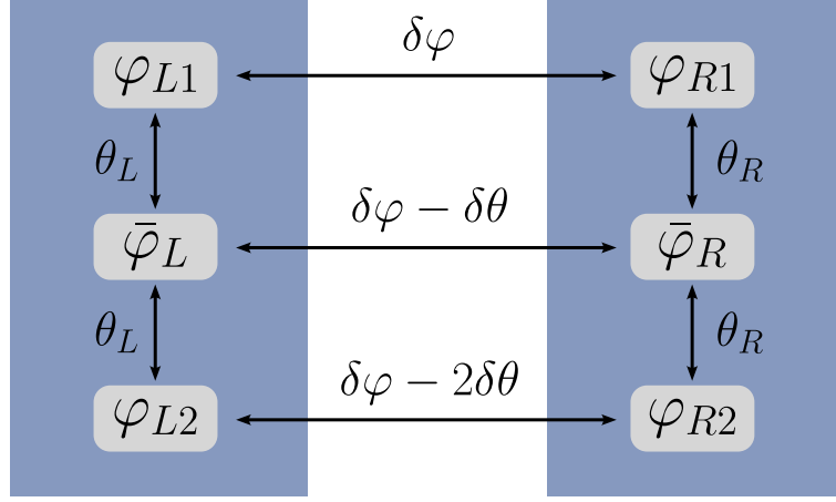
図 4.2 左右の超伝導位相と混成項位相
