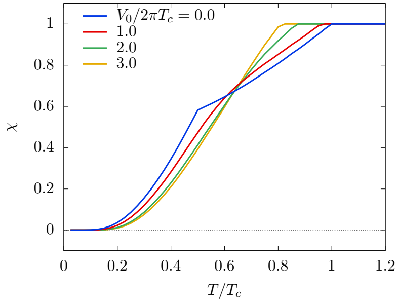
図 3.2 スピン磁化率の温度依存性
