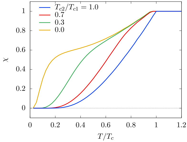
図 3.5 スピン磁化率の温度依存性
