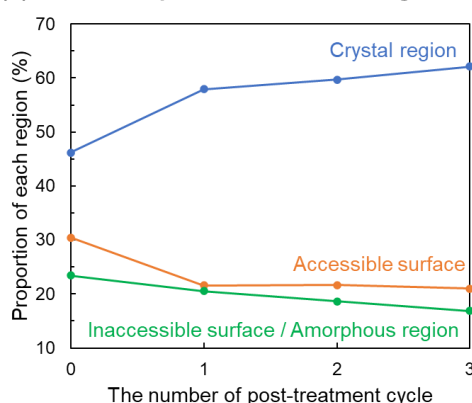
(d) Tensioned post-treatment on rayon
