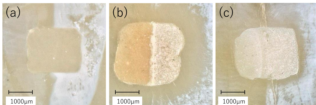
図3 脱灰後の試料表面のデジタルマイクロスコープ像。(a)GZF、(b)CDR、 (c)FIX。
