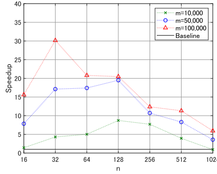
(b) OBCX (Cascade Lake)
