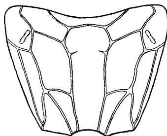
Fig. 3. Propodeum
