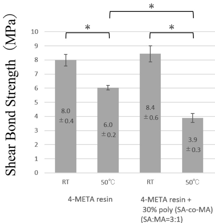
Fig.10 4-META レジン(4-META resin)、共重合比 3:1 の SA/MA 共重合ゲル添加 4-META レジン (4-META resin + 30%poly(SA-co-MA)(SA:MA=3:1)) の剪断強度 (* : p < 0.05 )
