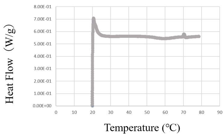
Fig.3 4META レジンの示差走査熱量測定
