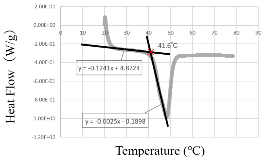
Fig.5 共重合比 3:1 の SA/MA 共重合ゲル添加 4META レジンの示差走査熱量測定
