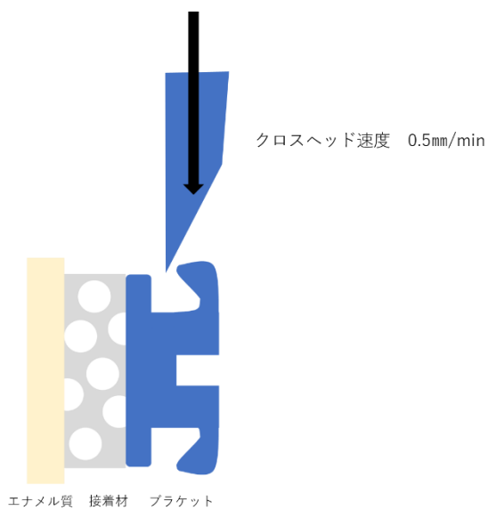
Fig.2 剪断試験の模式図
