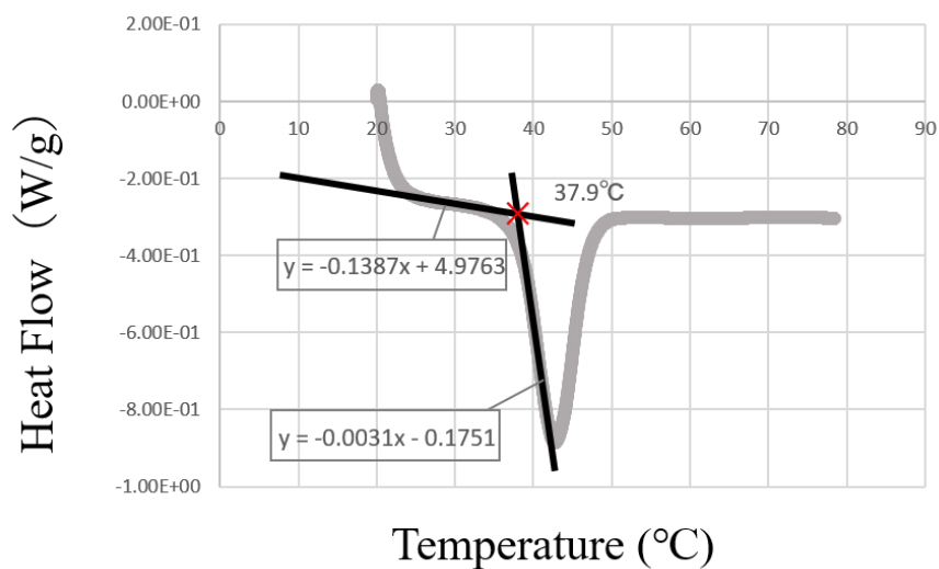
Fig.4 共重合比 1:1 の SA/MA 共重合ゲル添加 4META レジンの示差走査熱量測定
