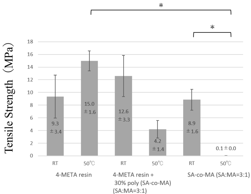
Fig.9 4-META レジン (4-META resin)、共重合比 3:1 の SA/MA 共重合ゲル添加 4-META レジン (4-META resin + 30%poly(SA-co-MA)(SA:MA=3:1))、共重合比 3:1 の SA/MA 共重合ゲル (SA-co-MA(SA:MA=3:1)) の引張強度 (* : p < 0.05 )
