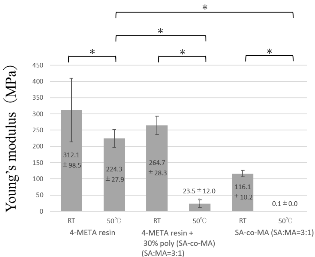
Fig.8 4-META レジン (4-META resin)、共重合比 3:1 の SA/MA 共重合ゲル添加 4-META レジン (4-META resin + 30%poly(SA-co-MA)(SA:MA=3:1))、共重合比 3:1 の SA/MA 共重合ゲル (SA-co-MA(SA:MA=3:1)) のヤング率 (* : p < 0.05 )
