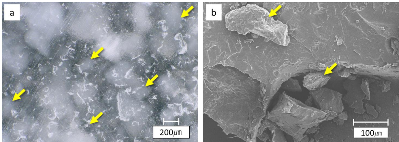
Fig.7 共重合比 3:1 の SA/MA 共重合ゲル添加 4 META レジンの顕微鏡像 a. 実体顕微鏡像 b. 走査電子顕微鏡像
