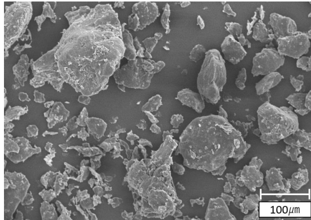
Fig.6 共重合比 3:1 の SA/MA 共重合ゲル粒子の走査電子顕微鏡像
