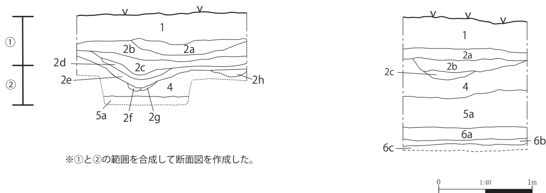
図 13 北キャンパス屋外パブリックスペース整備工事予定地の TP 180 断面図
