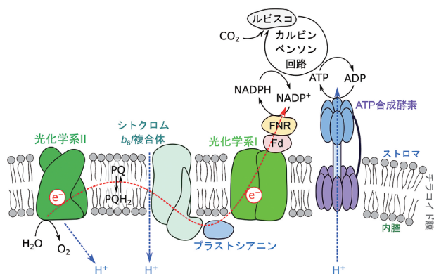
図1：酸素発生型光合成における直線的電子伝達とカルビン・ベンソン回路
