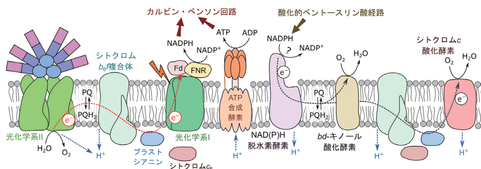
図4：光合成と呼吸の電子伝達が共存したシアノバクテリアチラコイド膜の模式図 直線的電子伝達および呼吸電子伝達をそれぞれ赤点線と黒点線で示す。
