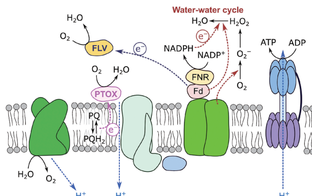
図2：本稿で述べた葉緑体における酸素還元反応の概要
