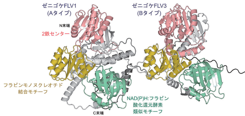
図3：ゼニゴケがもつAおよびBタイプFLVのAlphaFold予測構造
