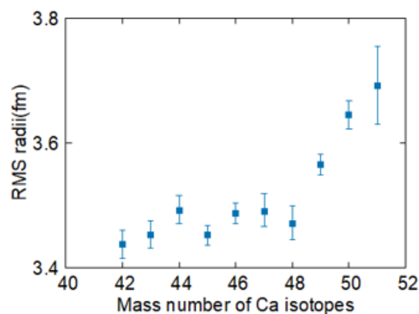
図 1.9 ^{42-51}\text{Ca} 同位体の平均二乗根半径 R_{rms}
