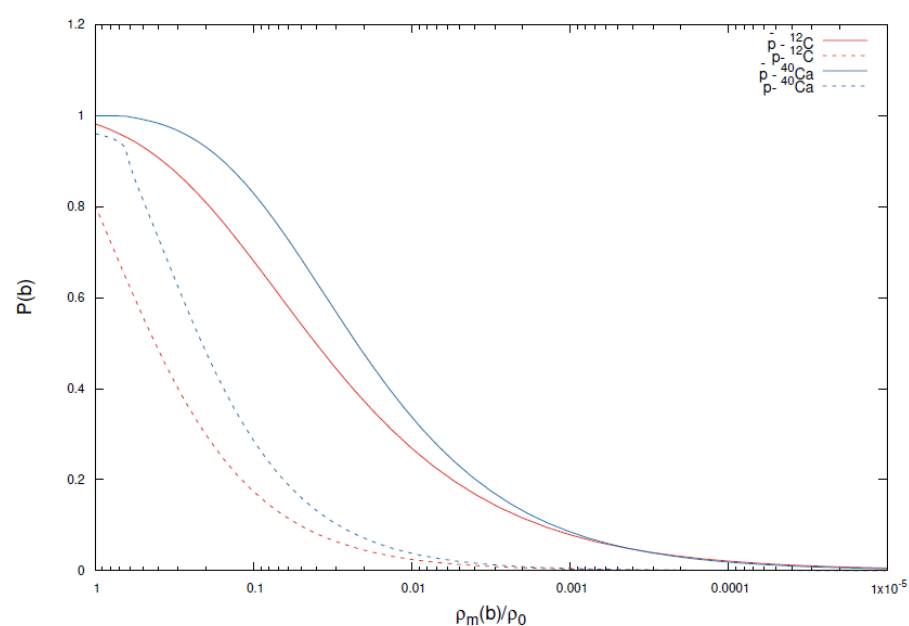
図 3.5 p(\bar{p})-^{12}\text{C} 、 p(\bar{p})-^{40}\text{Ca} の散乱について、反応率 P(b) と標的核の密度分布の中心密度に対する割合 \rho_m(b)/\rho_0 の関係。陽子散乱では中心密度の 1/10 程度、反陽子散乱では中心密度の 1/100 程度にまで感度があることが分かる。
