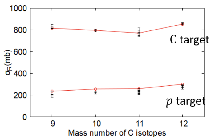
図 4.7 {}^9\text{--}{}^{11}\text{C} の p 散乱、 {}^{12}\text{C} 散乱の全反応断面積
