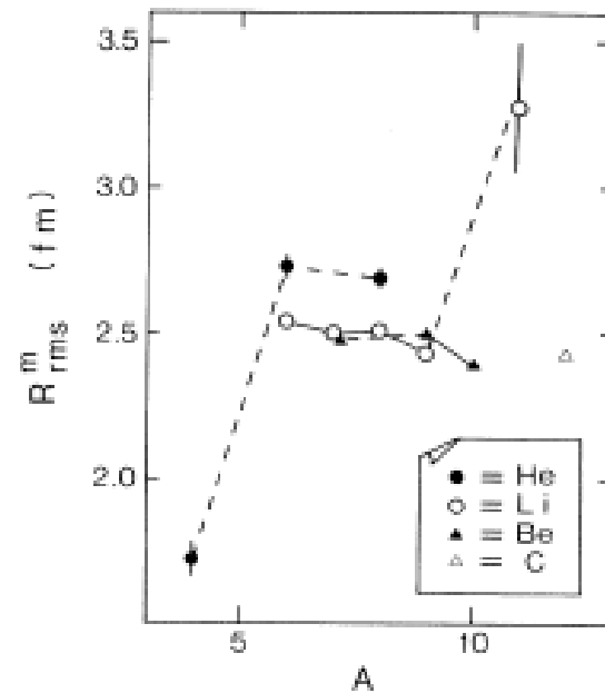
図 1.7 He、Li、Be、C 同位体の平均二乗根半径 R_{\text{rms}} ([1] より引用)
