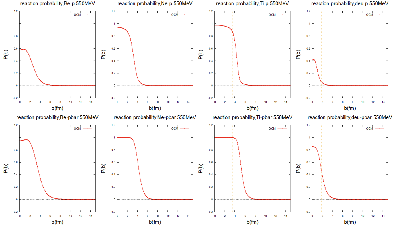
図 5.8 550MeV の ^8\text{Be} 、 ^{20}\text{Ne} 、 ^{44}\text{Ti} 、 d の p(\bar{p}) 散乱の反応率
