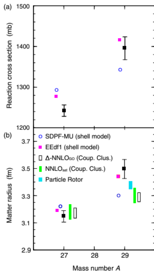
図 1.12 ^{27,29}\text{F} の全反応断面積およびそれより導出された物質半径 (黒四角形が [3] の実験結果。 [3] より引用)
