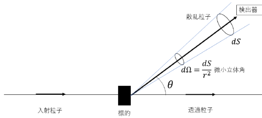
図 1.4 散乱実験の概略図。検出器により粒子の散乱の角度分布を観測する。
