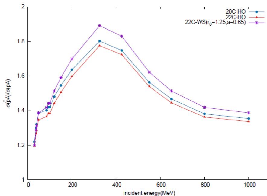
図 3.9 p(\bar{p}) - ^{20,22}\text{C} の散乱の全反応断面積比 \sigma_{R(\bar{p}A)}/\sigma_{R(pA)} 。Woods-Saxon (WS) ポテンシャルより求めた ^{22}\text{C} が調和振動子 (HO) 密度による ^{20,22}\text{C} と比べ大きな断面積比が得られた。
