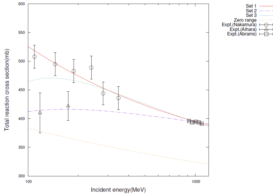
図 3.2 \bar{p}-^{12}\text{C} 散乱の全反応断面積の実験データ [8-10] と \beta_{\bar{p}N} が Set 1-3 及びゼロレンジの場合の計算。ゼロレンジでは実験データとは一致した結果は得られず、実験データを再現するように有限の \beta_{\bar{p}N} を定めた。
