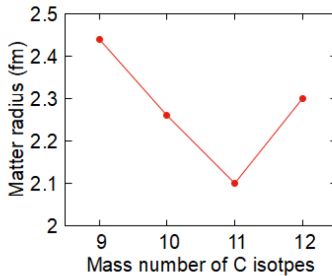
図 4.6 {}^9\text{--}{}^{11}\text{C} の物質半径
