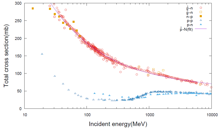
図 3.1 NN 、 N\bar{N} 散乱の全断面積の実験値
