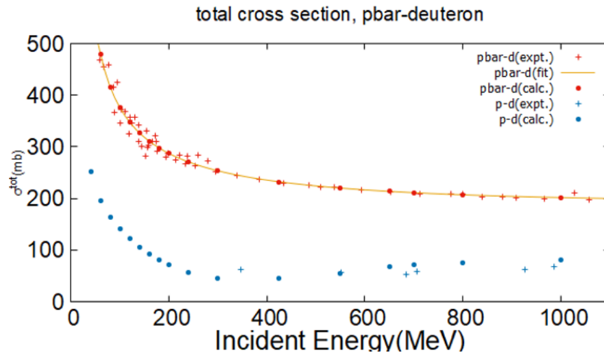
図 5.1 \bar{p} - d 散乱の全断面積
