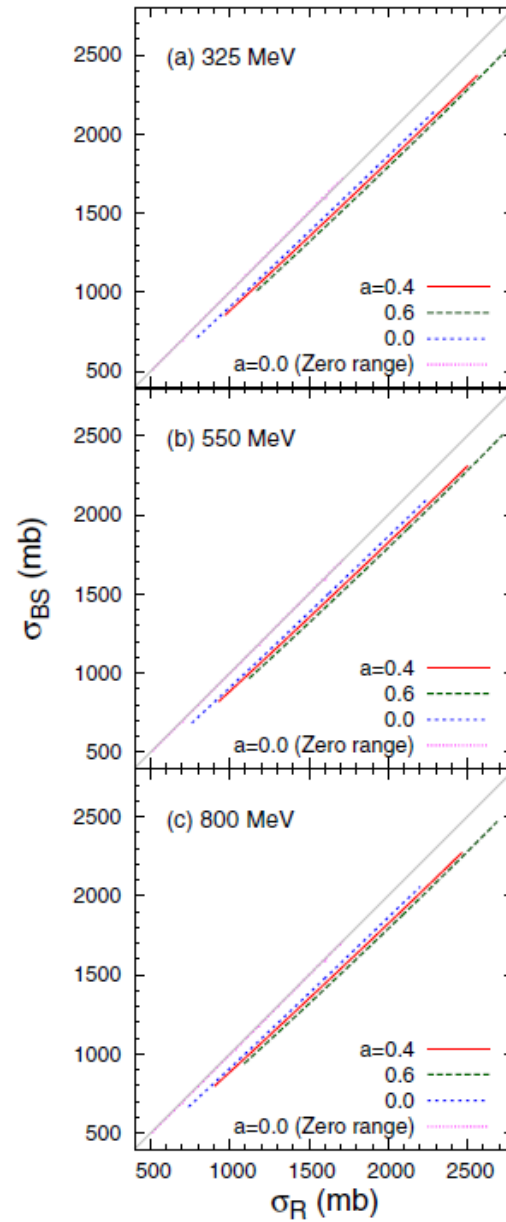
図 1.14 反陽子散乱における全反応断面積の黒球模型とのずれ ([17] より引用)
