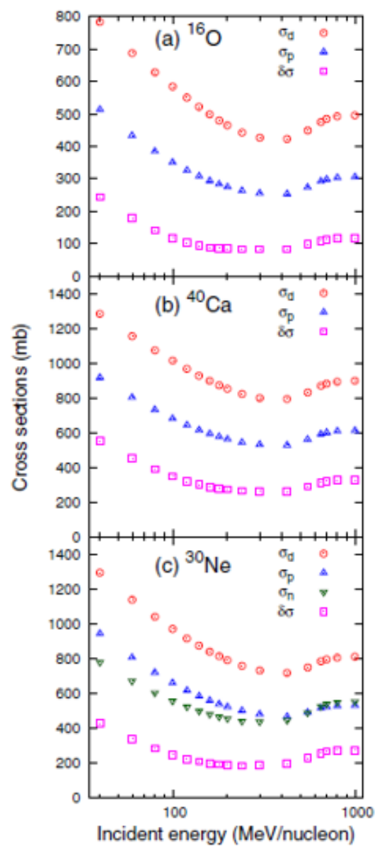
図 1.15 ^{16}\text{O} , ^{40}\text{Ca} , ^{30}\text{Ne} の全反応断面積。赤い丸は重陽子散乱、青の上向きの三角形は陽子散乱および ^{16}\text{O} , ^{40}\text{Ca} の中性子散乱、緑の下向きの三角形は ^{30}\text{Ne} の中性子散乱、マゼンタの四角形は陽子散乱と中性子散乱の和から重陽子散乱を差し引いたものである。いずれの原子核も重陽子散乱の全反応断面積は陽子散乱と中性子散乱のものの和よりも減少している事がわかる ([19] より引用)
