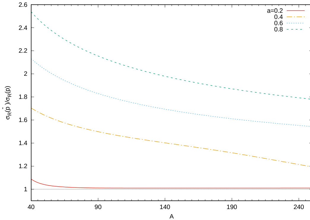
図 3.7 2pF 密度分布の原子核の散乱の \sigma_{R(\bar{p}A)}/\sigma_{R(pA)}
