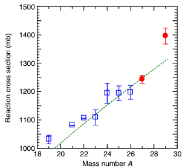
図 1.11 F 同位体の ^{12}\text{C} 散乱の全反応断面積。 ^{19-27}\text{F} では A^{2/3} の比例関係にあるところが、 ^{29}\text{F} ではそれを大きく外れて断面積が大きくなっている。( [3] より引用)
