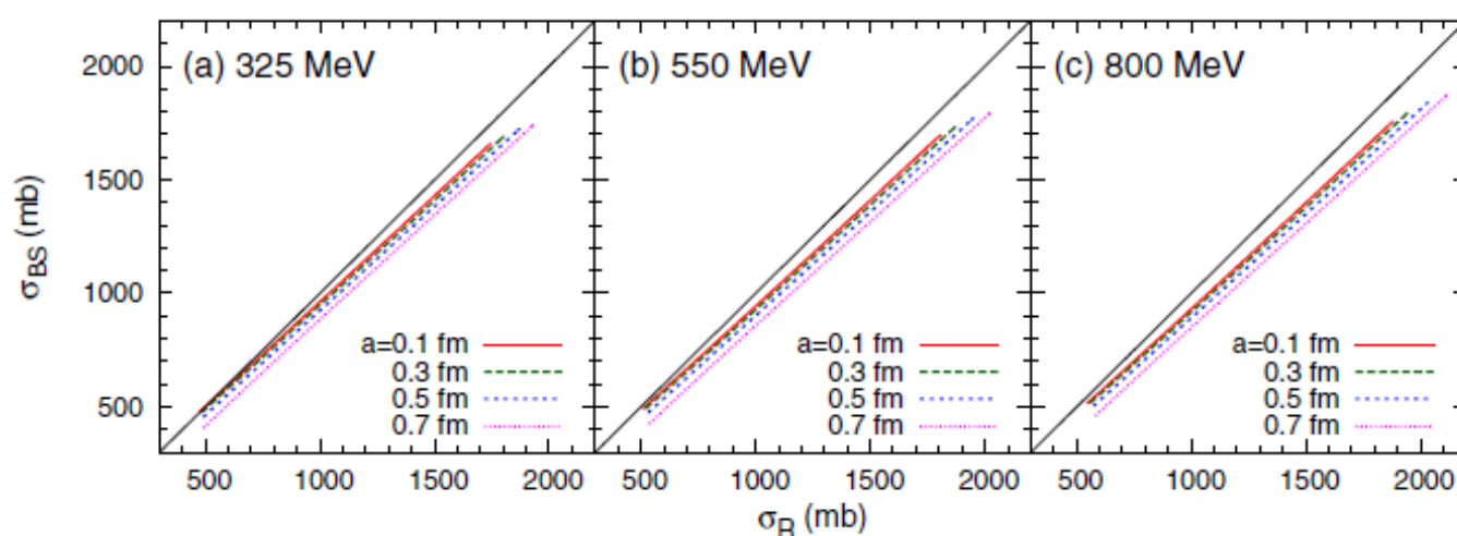
図 1.13 陽子散乱における全反応断面積の黒球模型とのずれ ([7] より引用)
