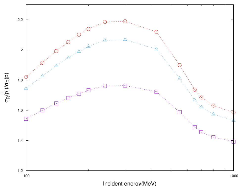
図 3.6 ^{12}\text{C} , ^{16}\text{O} , ^{40}\text{Ca} の原子核の散乱の \sigma_{R(\bar{p}A)}/\sigma_{R(pA)}
