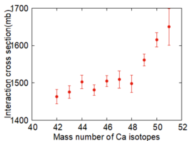
図 1.8 ^{42-51}\text{Ca} 同位体の相互作用断面積 \sigma_I
