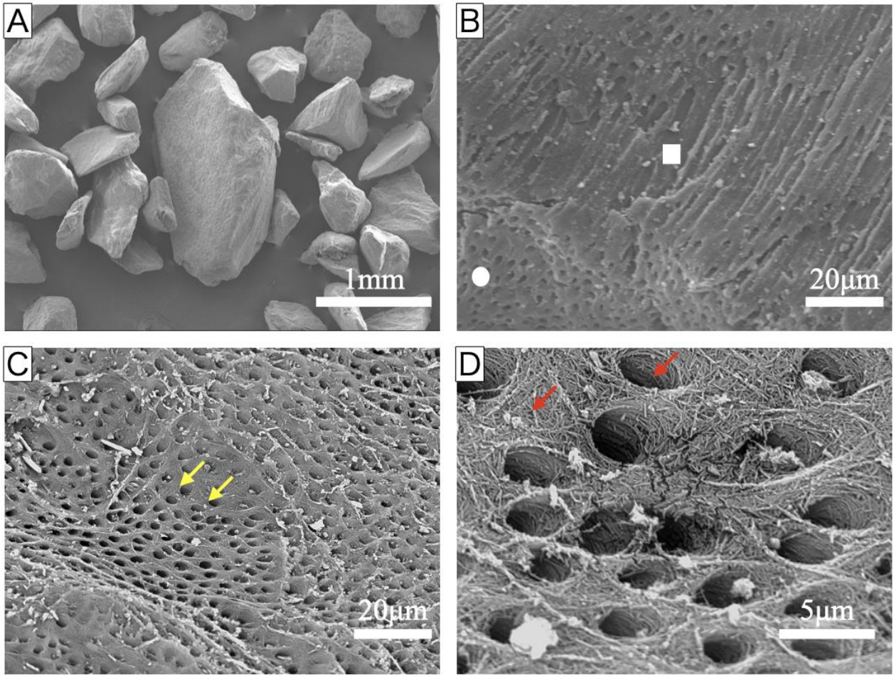
図3 BDDM の SEM 像
