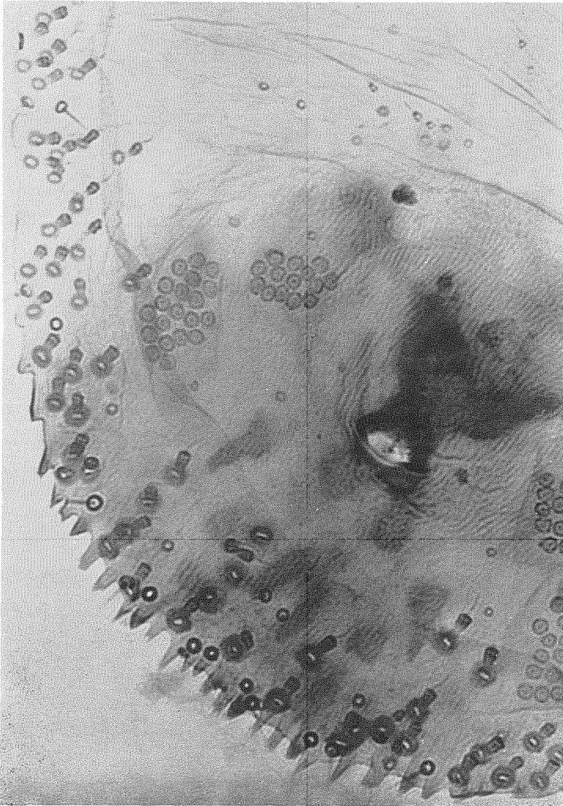
Fig. 3. Aleucaspis salla n. sp. Adult female: pygidium. 75NPL-27.
