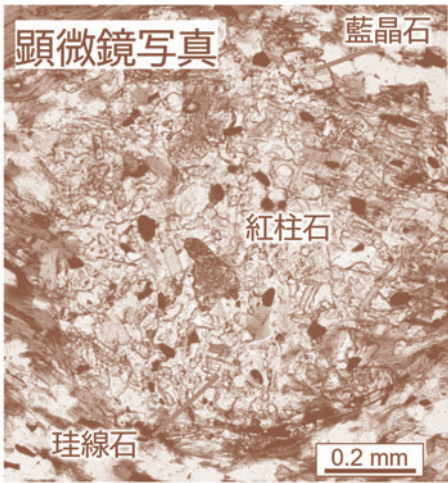
アルミノケイ酸塩鉱物3相(紅柱石、珪線石、藍晶石)すべてを含む変成岩の顯微鏡写真
