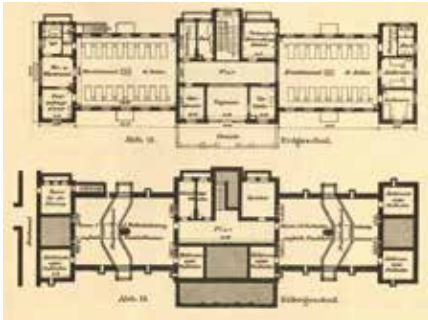
図 19 ザンクト・ゲオルク病院一般病棟平面図 (Ruppel, Das allgemeine Krankenhaus St. Georg in Hamburg 所載)
