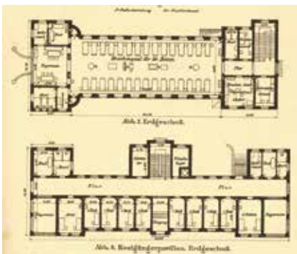
図 21 ザンクト・ゲオルク病院男性用外科病棟平面図 (Ruppel, Das allgemeine Krankenhaus St. Georg in Hamburg 所載)
