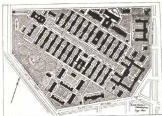
図15 ルドルフ・フィルヒョウ病院配置図 (Stevens, The American hospital of the twentieth century , 1921 所載)
