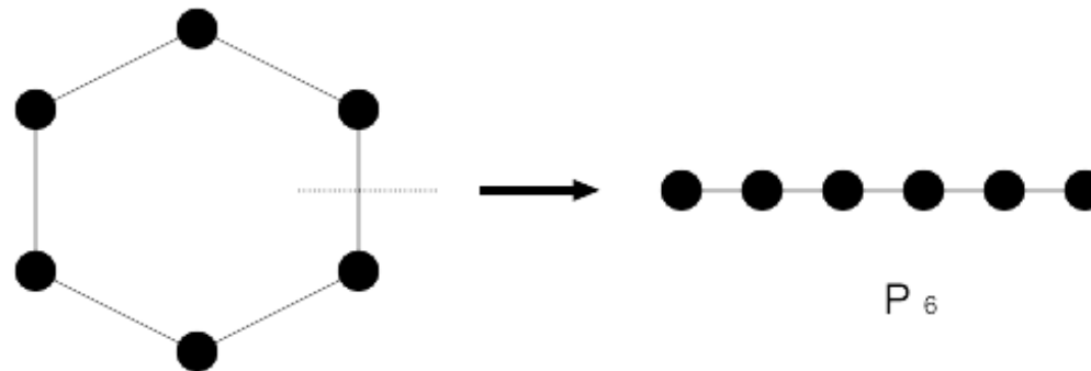
C_6
