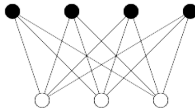
K_{4,3}
