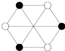
K_{3,3}
