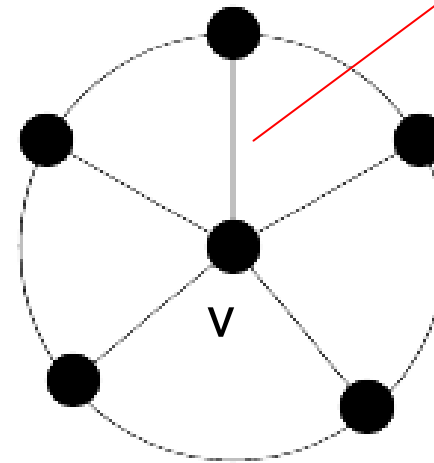
W_6
