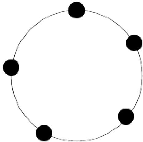
C_5
