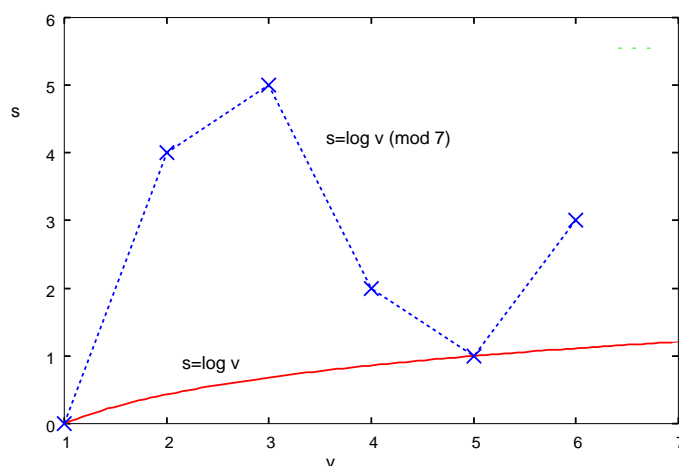
図 33: 離散対数 s = \log_a v \pmod{7} と底を a = 5 と選んだ場合の対数関数 s = \log_5 v 。離散対数の挙動は不規則である。
