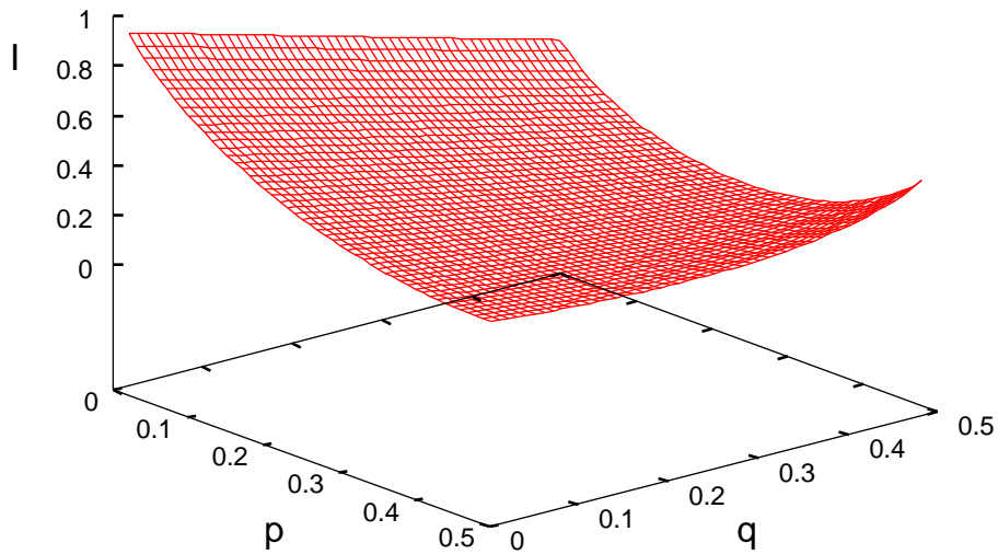
図 9: この問題で扱う通信路の相互情報量 I . p, q はそれぞれ [0, 0.5] の間でプロットしてある. q = 0 のとき, I は p = 1/2 で最小値をとる ( I は p = 1/2 の軸に関して対称であることに注意).
